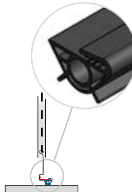
Junta de lámina final
