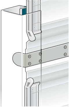
Opción ganchos antitormenta
