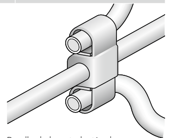
Detalle de la articulación de seguridad patentada para las persianas tipo TUBONDA R.
