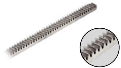
CRM72 Cremallera 22x22x2000 cincada de hierro
